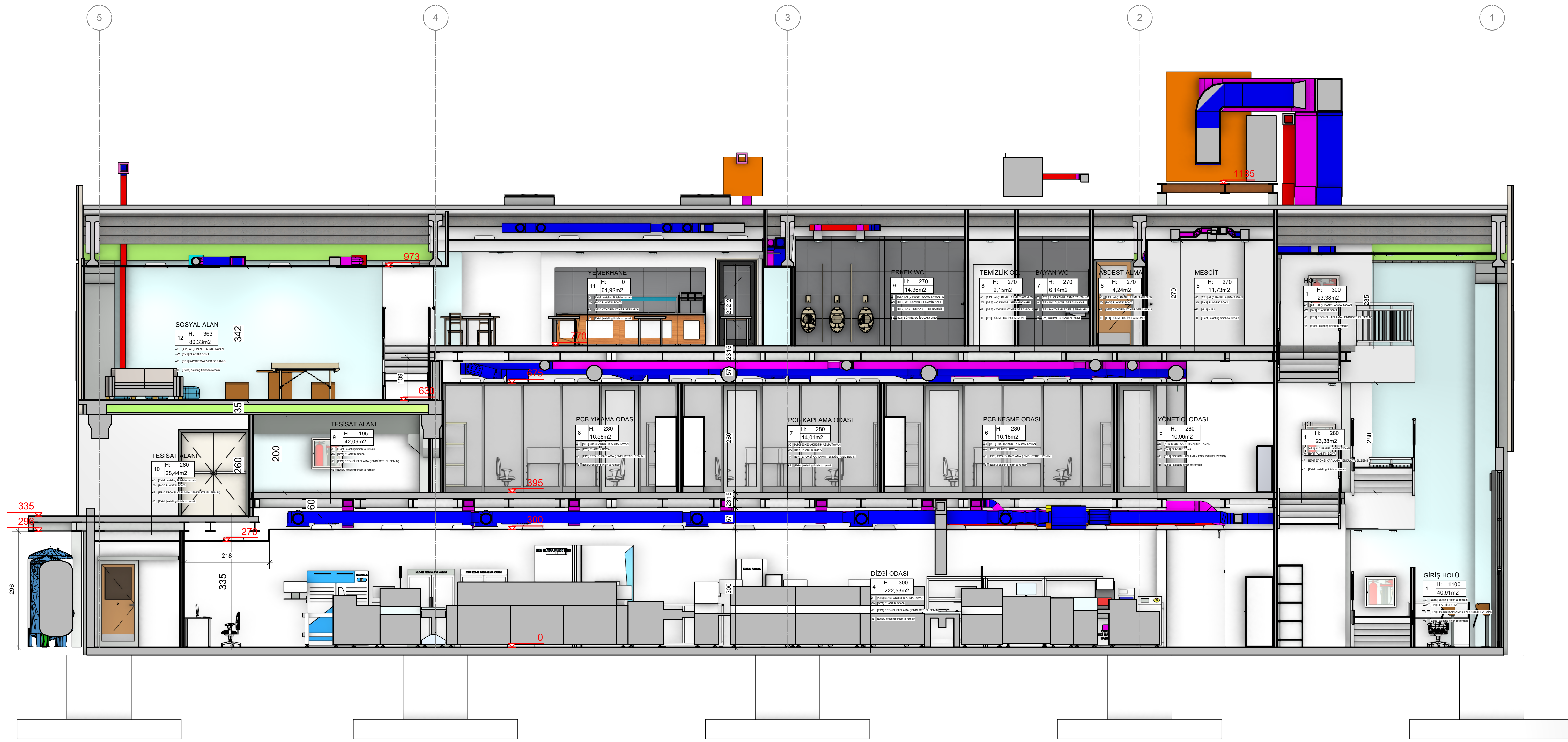
2 2-2 KESİTİ Scale: 1:50
