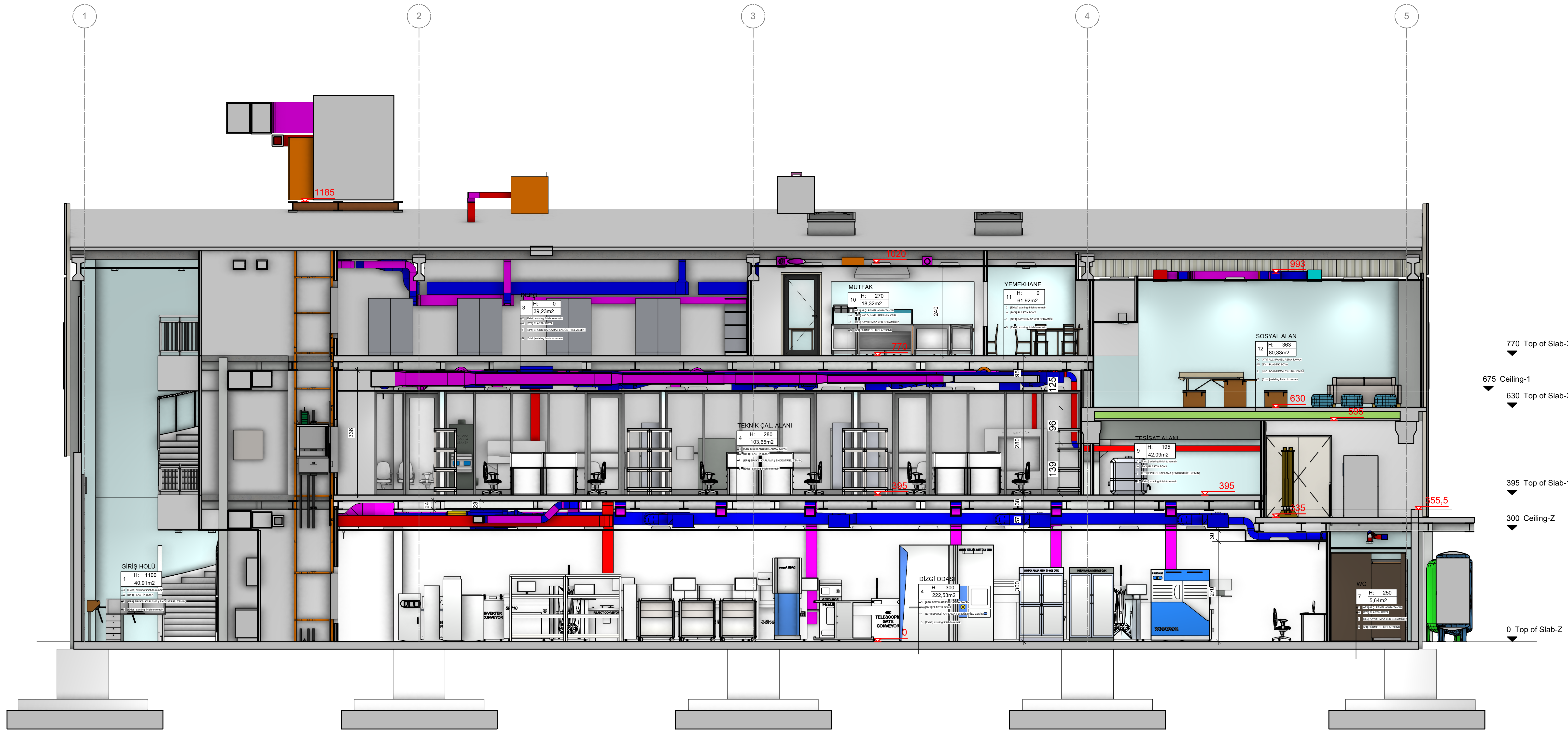
1 1-1 KESİTİ Scale: 1:50
